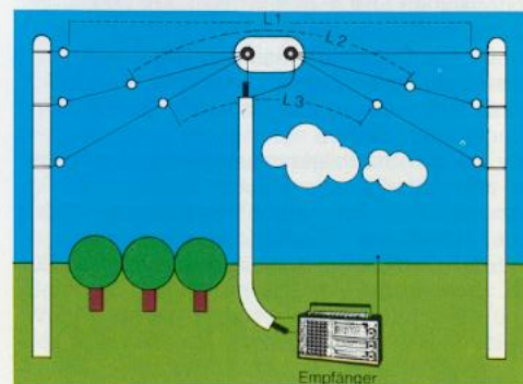
Mehrbandantenne
