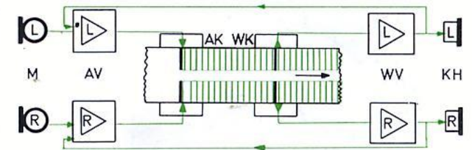
Echo-Aufnahme (Stereo)
