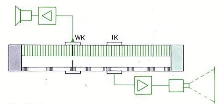
Dia-Vertonung
