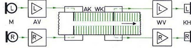
Hinterbandkontrolle (Stereo)
