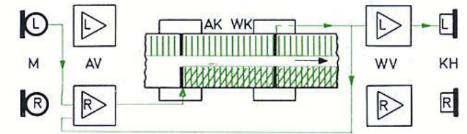
Multi-Playback 2. Aufnahme
