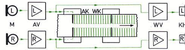
Mithören (Stereo)
