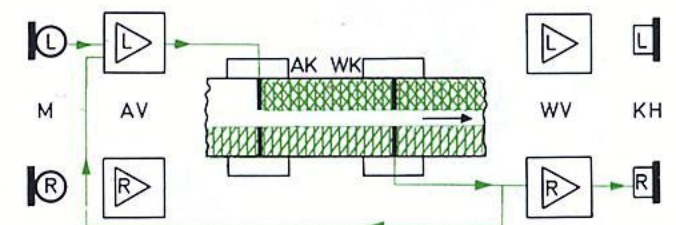
Multi-Playback 3. Aufnahme
