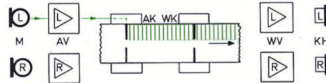
Synchron-Playback 1. Aufnahme
