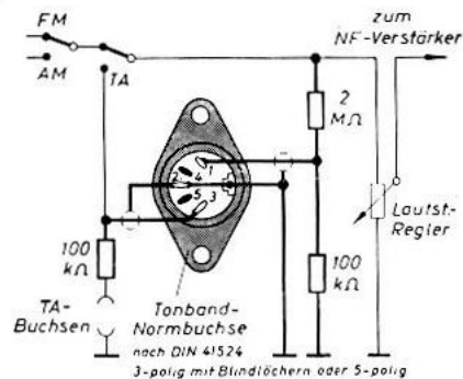
Abb. 2 Blick auf die Lötanschlüsse der Buchse
