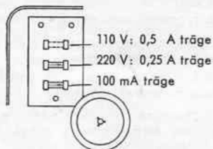
TK 24-Chassis von oben gesehen
