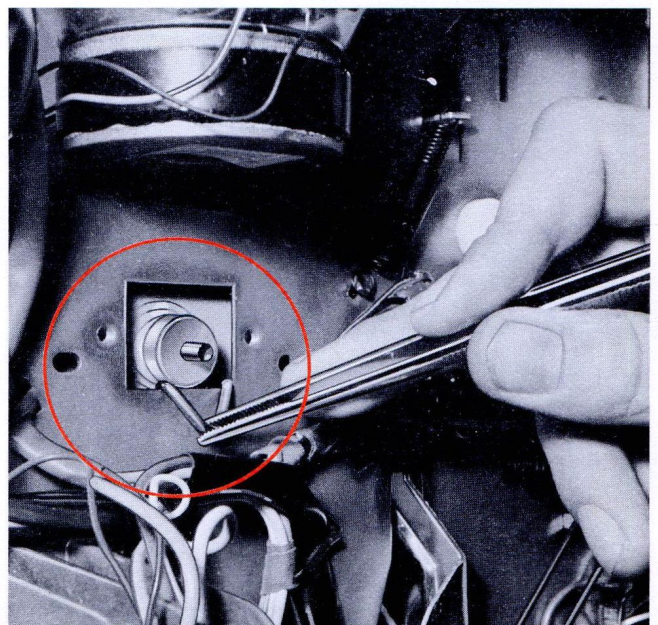
Abb. 7 Riemenwechsel bei abgeschraubtem Tonwellenlager
