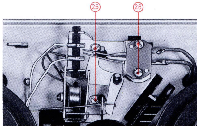
Abb. 15 Einstellen der Abschaltautomatik
