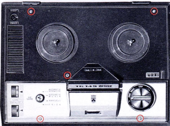
Abb. 2 Vier Schrauben halten den gesamten Aufbau
