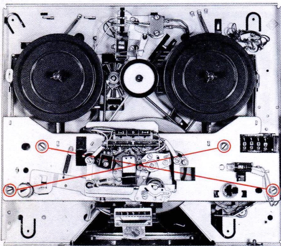
Abb. 3 Entfernen des Bodens
