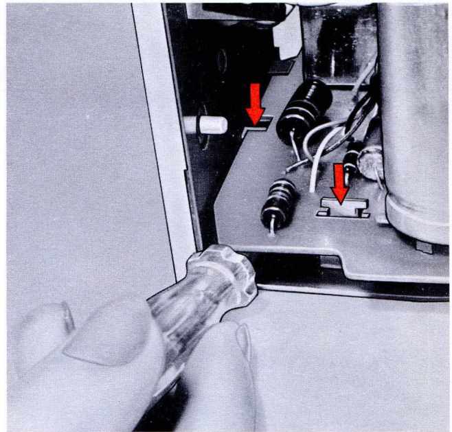
Abb. 5 Aushängen der Druckplatte
