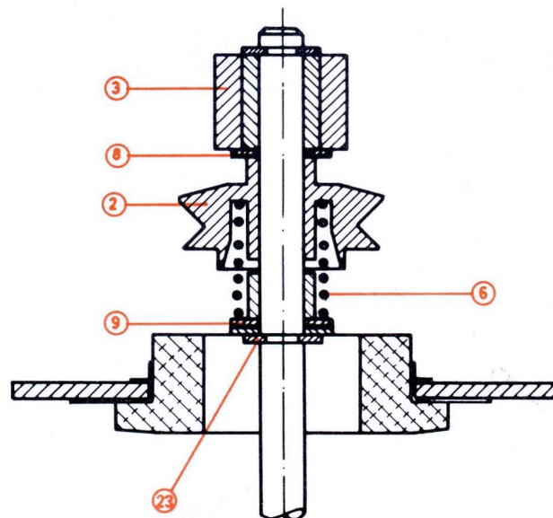
Abb. 10 Antrieb ohne Lüfter und Überlastungssicherung
