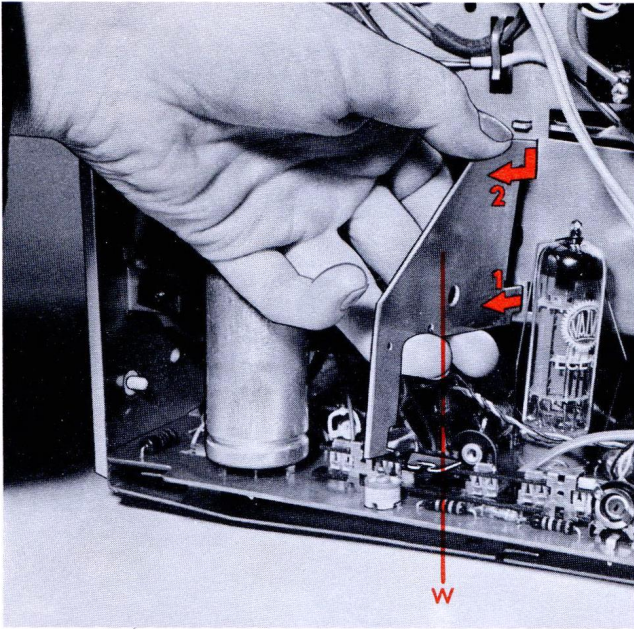
Abb. 4 Herausheben des Winkelhebels
