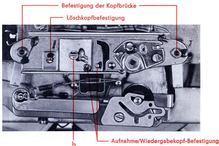
Abb. 16 Köpfe bei Halbspurgeräten
