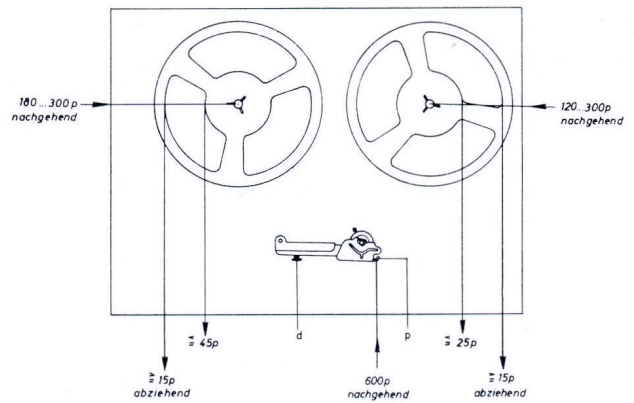
Abb. 12 Mechanische Meßpunkte
