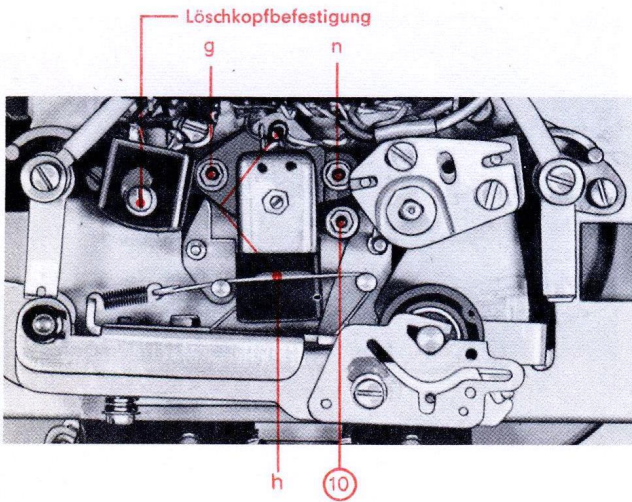
Abb. 18 Köpfe bei Viertelspurgeräten
