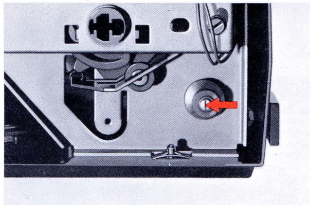
Abb. 14 Befestigungspunkt der Antriebsteile bei U-Geräten und 60 Hz Umbau
