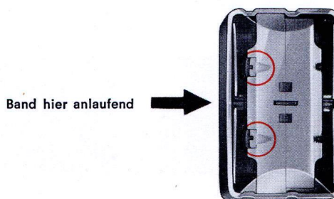
Abb. 17 Aufnahme/Wiedergabekopf Einbau
