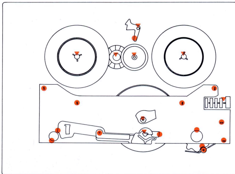
Abb. 8 Schmierplan
