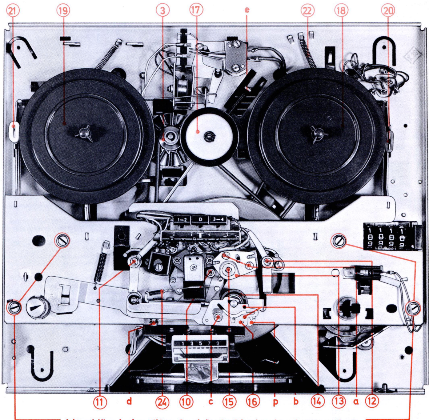
Abb. 11 Gesamtabbildung TK 145 de luxe
