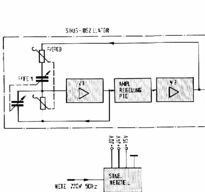
Abb. 1: Blockscha bild
