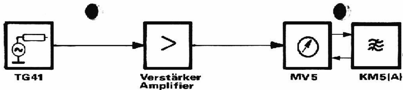
Abb. 6: Meßanordnung zur Prüfung des Klirrfaktors
