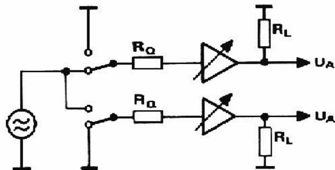
Abb. 4: Anordnung zum Messen des Übersprechens
