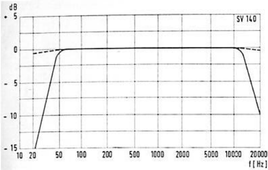
Efficacité du filtre combiné. Délimitation de la plage de transmission de 40 à 12 500 Hz.
