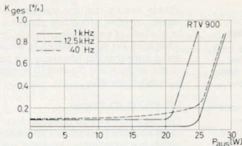
Klirrfaktorkurven Taux de distortion Fattore di distorsione
