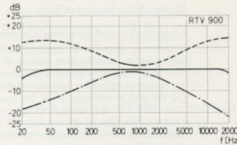
Wirkungsbereiche der Klangregler Effective range of tone controls Plages d'action des réglages de tonalité Campo d'azione dei regolatori di tono
