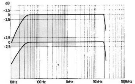
Frequenzgang TA-Magnet (über Schneidkennlinien-Nachbildung) mit steilem Abfall der Frequenzen unterhalb 40 Hz, gemessen am Lautsprecherausgang.
