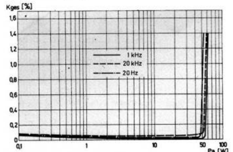
Klirrfaktor in Abhängigkeit von der Ausgangsleistung
