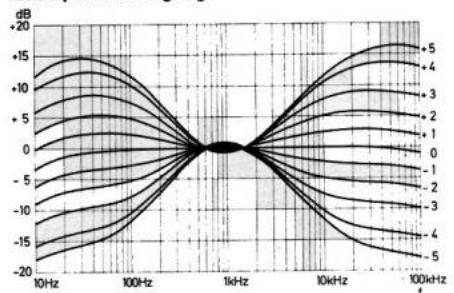
Wirkungsbereich der Baß- und Höhensteller über Meßeingang TB 1, gemessen am Lautsprecherausgang.
