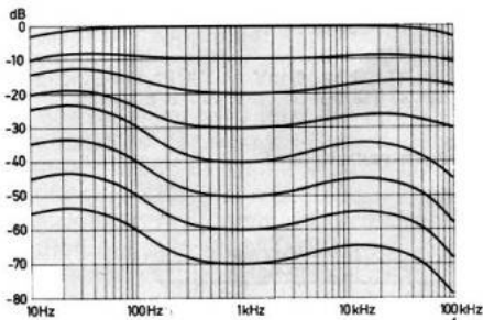
Verlauf der gehörrichtigen Lautstärkekorrektur (Contour).
