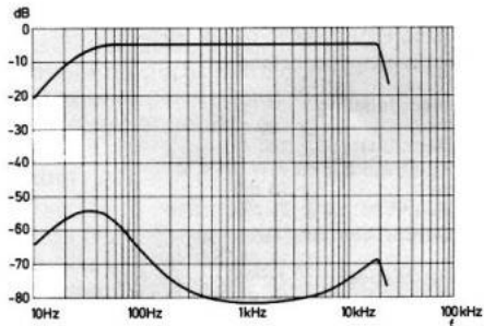
Obersprechdämpfung L→R/R→L, gemessen über Schneidkennlinien-Nachbildung (Meßeingang TA-Magnet).
