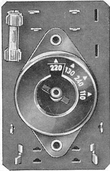
Netzspannungswähler am Rundfunkchassis
