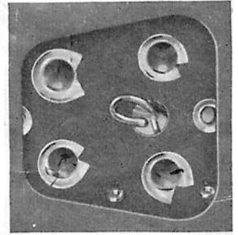
Anschlußbuchsen für UKW-Dipol, Erde und Antenne
