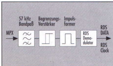
RDS-Modul.
