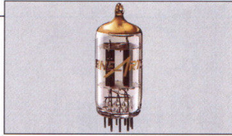
Hochwertige Spanngitterröhren E 83 CC.
