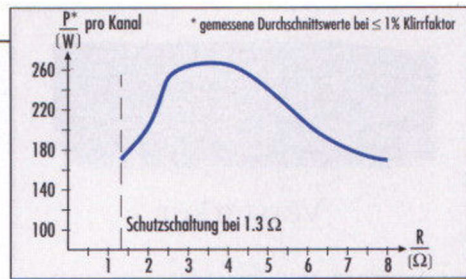
Ausgangsleistung A-9009.
