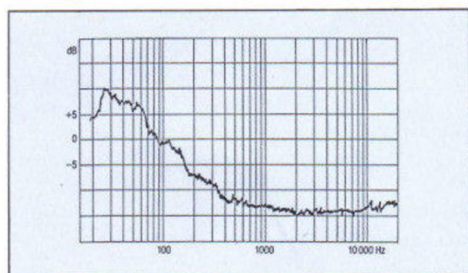
Wiedergabe-Fremdspannung mit Schnittbandkern.
