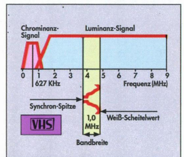
Signalverlauf bei VHS
