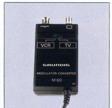
Modulator M 60 für Camera-Recorder S-VS- C 80, VS-C 60 und VS-C 40.
