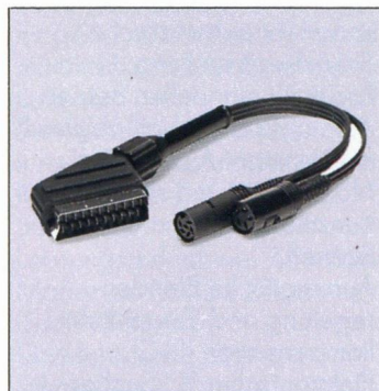
Euro-AV-Kabel VK 32a Verbindung von Grundig Video-Recorder mit DIN-AV- Buchse und Grundig Farb- fernseher mit Euro-AV-Buchse, 0,2 m lang.
