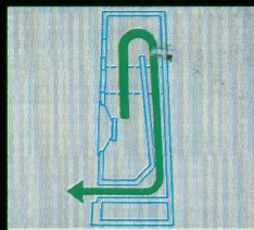
Weg der rückwärtigen Schallenergie durch den Transmissionline-Ionkanal.
