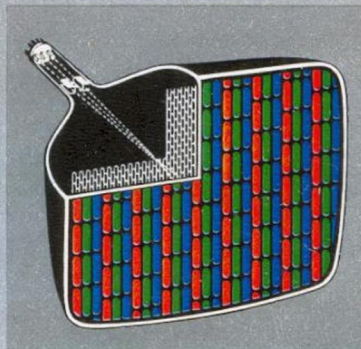
Brandneue Schlitzmasken-Bildröhre
