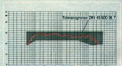
HiFi-Box 203 M Frequenzgang, gemessen nach DIN 45500 Bl. 7 mit Terzrauschen
