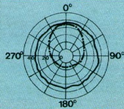
Abstrahlung im schalltoten Raum: ----- Normaler Hochton-Lautsprecher ———— Grundig-HiFi-Kugelstrahler
