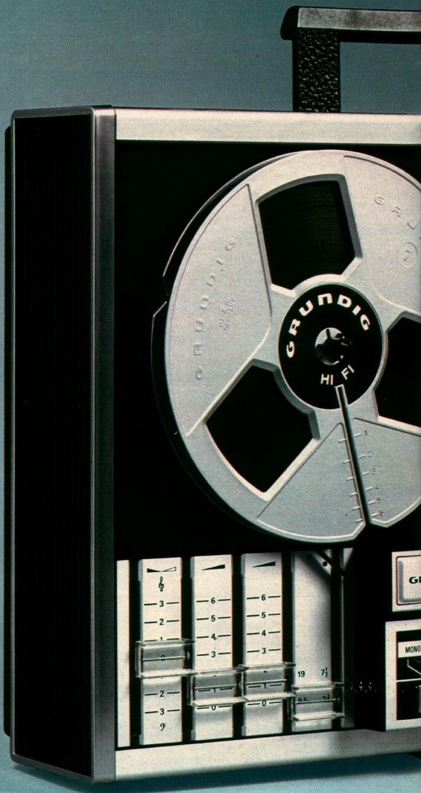
1 Die moderne Einknopfbedienung für alle Funktionen. 2 Großes, beleuchtetes Aussteuerungs-instrument in %- und dB-Eichung. 3 Bedienungselemente Spurumschaltung.
