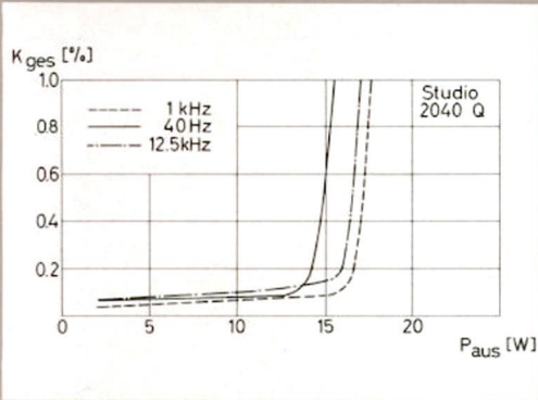
Klirrfaktor bei verschiedenen Frequenzen
