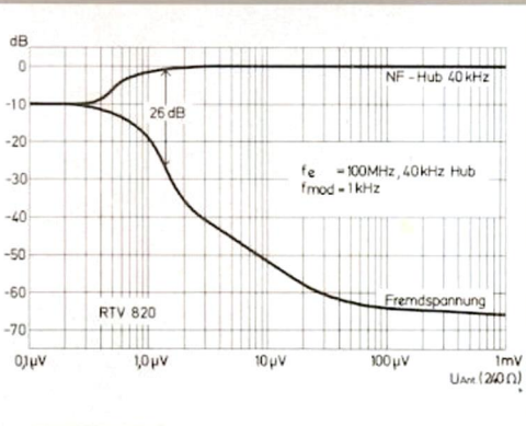
FM-Signal- und Fremdspannungsverlauf in Abhängigkeit von der Antennenspannung.
