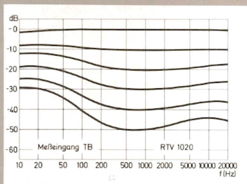
Verlauf der gehörrichtigen Lautstärkeregelung (Contour)
