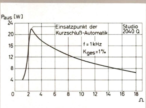
Ausgangsleistung bei verschiedenen Abschlußwiderständen
