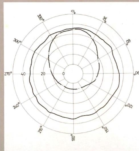
Abstrahlung im schalltoten Raum - - - normaler Hochton-Lautsprecher — GRUNDIG HiFi-Kugelstrahler
