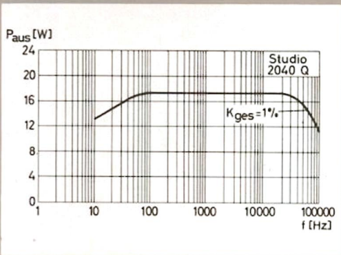
Leistungsbandsbreite
