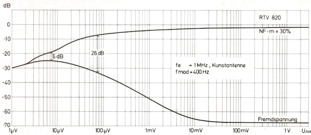
AM-Signal- und Fremdspannungsverlauf in Abhängigkeit von der Antennenspannung.
