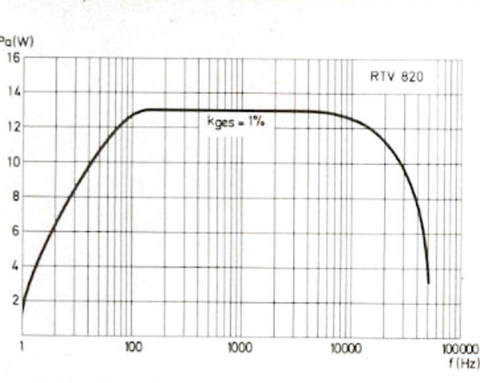
Leistungsbandbreite
