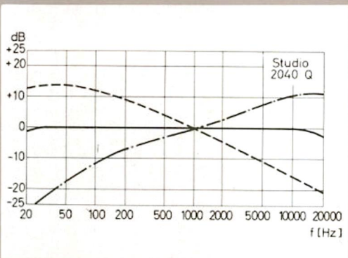
Wirkungsbereich der Klangregler
