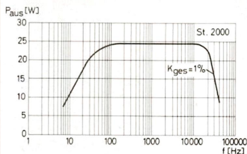
Leistungsbandbreite
