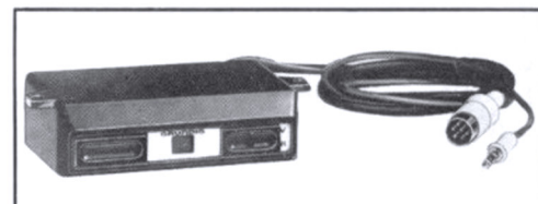
Verkehrs-Rundfunk-Decoder VD 3 Speziell für den Weltklang 4800. Für Montage unter dem Armaturenbrett (w. VD 2). Nach Umschalten des Schiebeschalters sucht der „Statomat“ nur Stationen, die Verkehrs- rundfunk-Programme ausstrahlen. Mit einer zusätzlichen Taste kann außerdem der Suchlauf direkt am VD 3 betätigt werden – Sie brauchen also nicht die Statomat-Taste des Autosupers zu drücken. Abmessungen: 114 x 35 x 70 mm (B x H x T) unverbindliche Preisempfehlung mit MWSt.: DM 70.-
