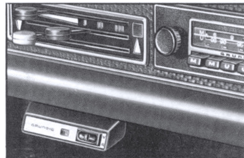
Verkehrs-Rundfunk-Decoder VD 2 Für Montage unter dem Armaturenbrett. Befes- tigung mit 2 Schraubtaschen. Funktionen im Prinzip wie bei VD 1. Abmessungen: 114 x 35 x 70 mm (B x H x T) unverbindliche Preisempfehlung mit MWSt.: DM 60.-
