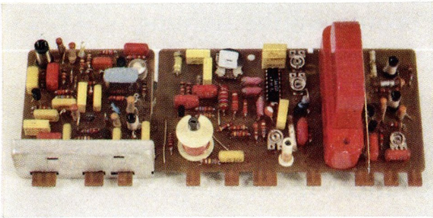
Farbteil mit integrierten Schaltkreisen
