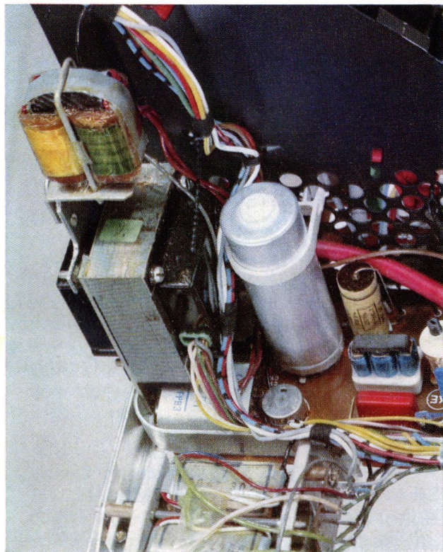
Ausschnitt aus Netzteil und stabilisierter Bildröhrenheizung
