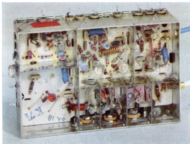
Vollelektronischer Allbereich-Tuner
