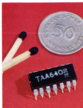
1 Vollintegrierter Schaltkreis für Ton-ZF und FM-Demodulator
