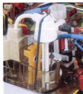
2 Selen-Hochspannungsgleichrichter für hohe Trennschärfe
