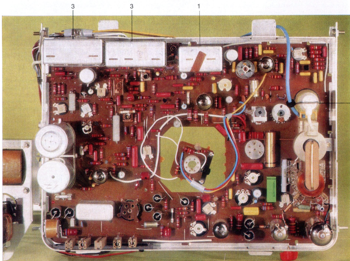
3 4stufiger Bild-ZF-Verstärker
