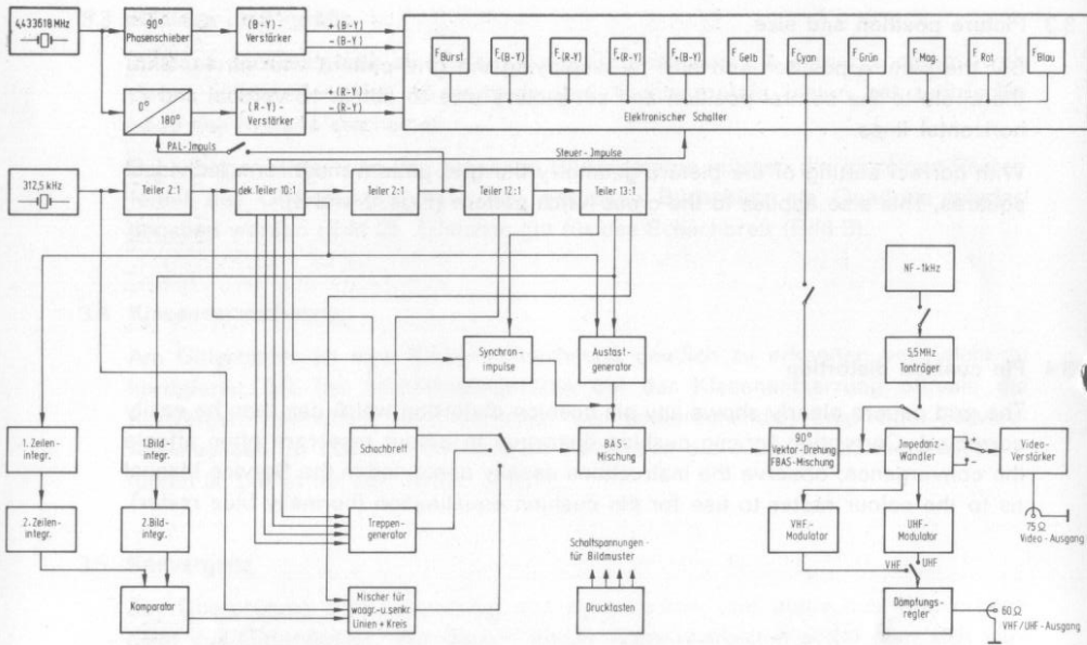
Bild 1: Blockschaltbild des FG 5
