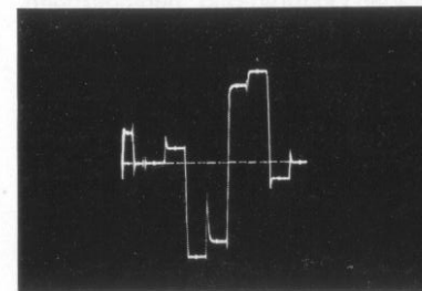
Bild 6a: (R-Y)-Auszug des Normtest- bildes
