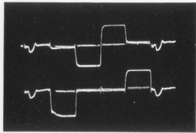
Bild 16: Oszillogramm des Sondertest- bildes bei richtigem Empfängerabgleich Fig. 16: Oscillogram of special test pattern with correctly aligned receiver
