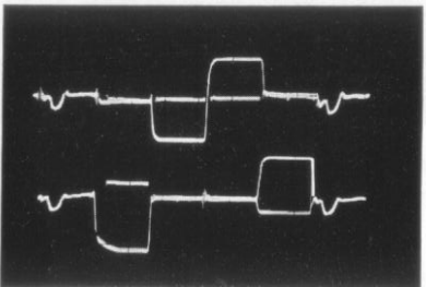
Bild 18: Oszillogramm des Sondertest- bildes bei verstimmtem 90°-Glied im (B-Y)-Synchrodemodulator Fig. 18: Oscillogram of special test pattern with de-tuned 90° network in the (B-Y) synchron. demodulator
