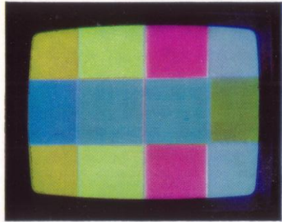
Bild 9: Sondertestbild bei verstimmtem 90°-Glieder im (B-Y-Synchr.-Demodulator)
