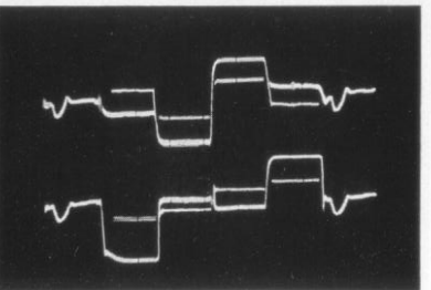
Bild 19: Oszillogramm bei Fehl- abgleich von PAL-Decoder und Allgemein- phase Fig. 19: Oscillogram with incorrectly set PAL decoder and general phase.
