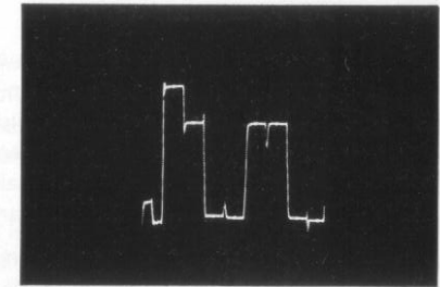
Bild 5a: R-Auszug des Normtestbildes
