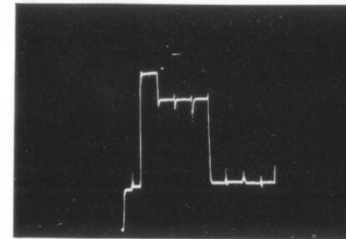
Bild 5b: G-Auszug des Normtestbildes
