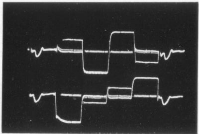
Bild 17: Oszillogramm des Sondertest- bildes bei falschem Abgleich des PAL- Decoders Fig. 17: Oscillogram of special test pattern with incorrectly aligned PAL decoder
