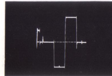
Bild 14: Demoduliertes (R-Y)-Signal Fig. 14: Demodulated (R-Y)
