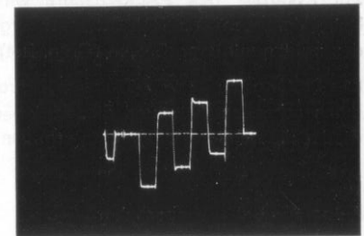
Bild 6b: (B-Y)-Auszug des Normtest- bildes
