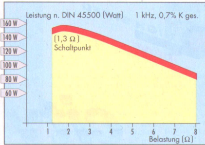
Rauscharme Eingangsimpedanz-Wandlerstufe Leistungsdiagramm in Abhängigkeit von der Belastung
