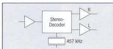
Absolute Stereo-Kanaltrennung durch Keramik-Resonatoren im PLL-Stereodecoder.
