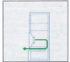
Weg der rückwärtigen Schallenergie durch den Transmissionline-Tonkanal.
