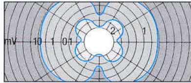
1: Magn. Streufeld bei üblichem Trafo. 2: Magn. Streufeld bei Schnittbandkern-Trafo.
