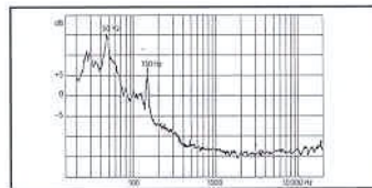
Wiedergabe-Fremdspannung mit herkömmlichem Trafo.
