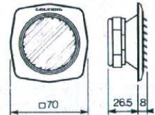
L/U 29 50 Watt. Hochton-Lautsprecher (Tweeter). Nur in Verbindung mit einem Baß- oder Breitbandlautsprecher (z. B. L/U 26b etc.) verwendbar. Übertragungsbereich 3 000... 25 000 Hz.
