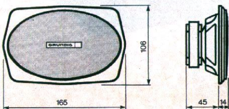
L/U 27 50 Watt. Übertragungsbereich 60... 16 000 Hz.
