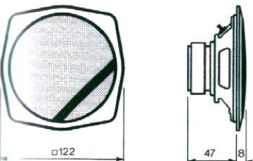
L/U 24a 40 Watt. Übertragungsbereich 60... 14000 Hz.
