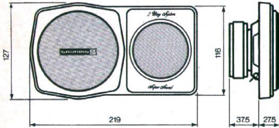
L/U 30a 30 Watt. Zweiweg-Lautsprecher Übertragungsbereich 60... 25 000 Hz.
