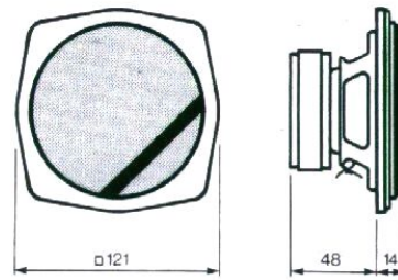
L/U 25a 50 Watt. Übertragungsbereich 60... 14000 Hz.
