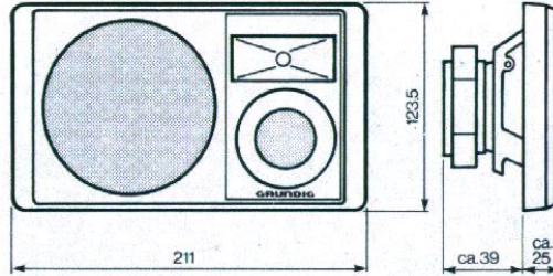
L/U 33 50 Watt. Dreiweg-Lautsprecher Übertragungsbereich 60... 22 000 Hz.
