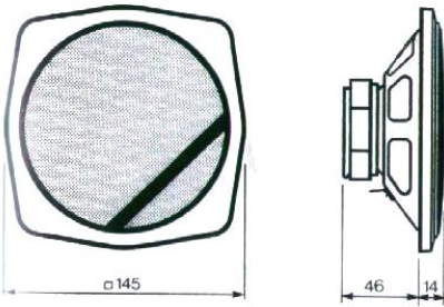
L/U 26b 50 Watt. Übertragungsbereich 60... 16000 Hz.
