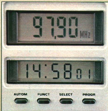
1. 6 UKW-Programmtasten – fest programmierbar. 2. LCD-Frequenzanzeige und LCD-Quarz-Schaltuhr
