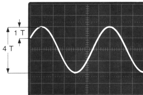
Amplitude = 4 Teile Triggerpegel = 1 Teil gleich \frac{1}{4} der Gesamtamplitude
