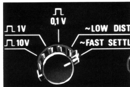
Betriebsartenschalter Stellung LOW DIST.: Kleiner Klirrfaktor FAST SETTL.: Schnelle Einschwingzeit bei Frequenzänderung
