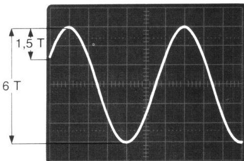
Amplitude = 6 Teile Triggerpegel = 1,5 Teile gleich \frac{1}{4} der Gesamtamplitude
