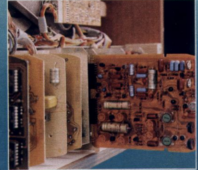
Multi-Modultechnik mit 12 steckbaren Baugruppen
