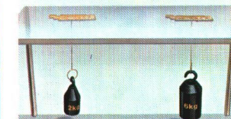
Normale Technik Belastet man die normale Leiterplatte mit 6 kg, so wird die Lötverbindung Bauelement/Leiterplatte in Bruchteilen einer Sekunde zerstört. Die Leiterplatte in LL-Technik dagegen trägt 6 kg spielend!
