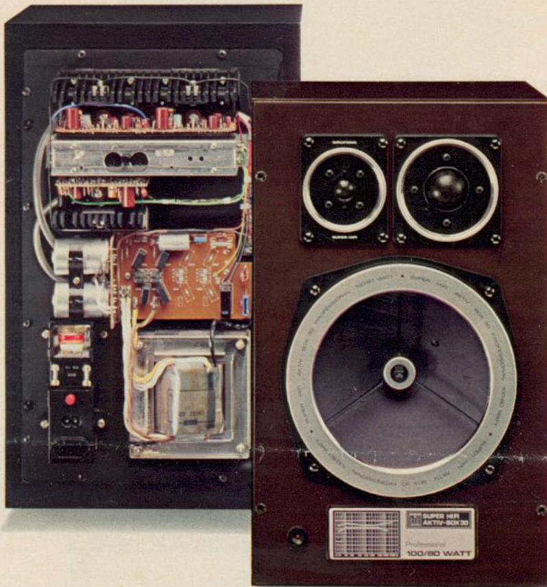
Aktiv-Boxen 30
