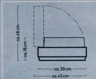
1. Skizze Studio 2000 2. Drehfußgestelle für alle Studios Siehe Zubehör Seite 113
