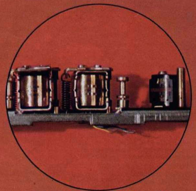
Hinterbandkontrolle und Echo durch Drei-Kopf-Anordnung.
