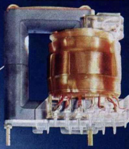
Zellentransformator
