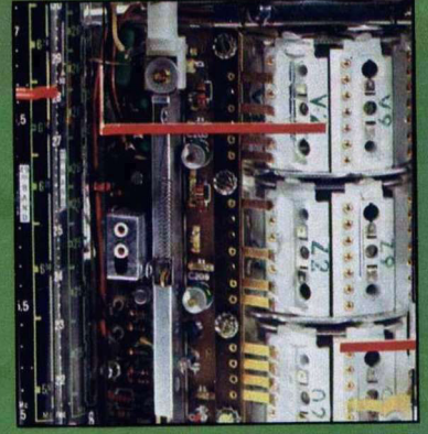
Kurzwellen-Trommeltuner des Satellit 1000 mit doppelter Bandspreizung (KW 2 bis KW 9).
