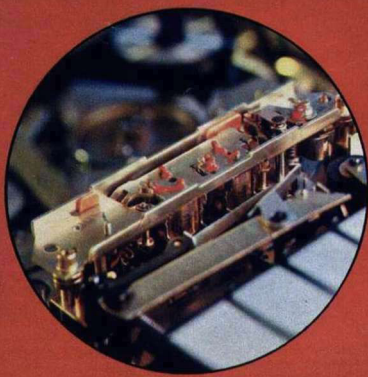
Vier-Kopf-Anordnung beim TK 600 d.
