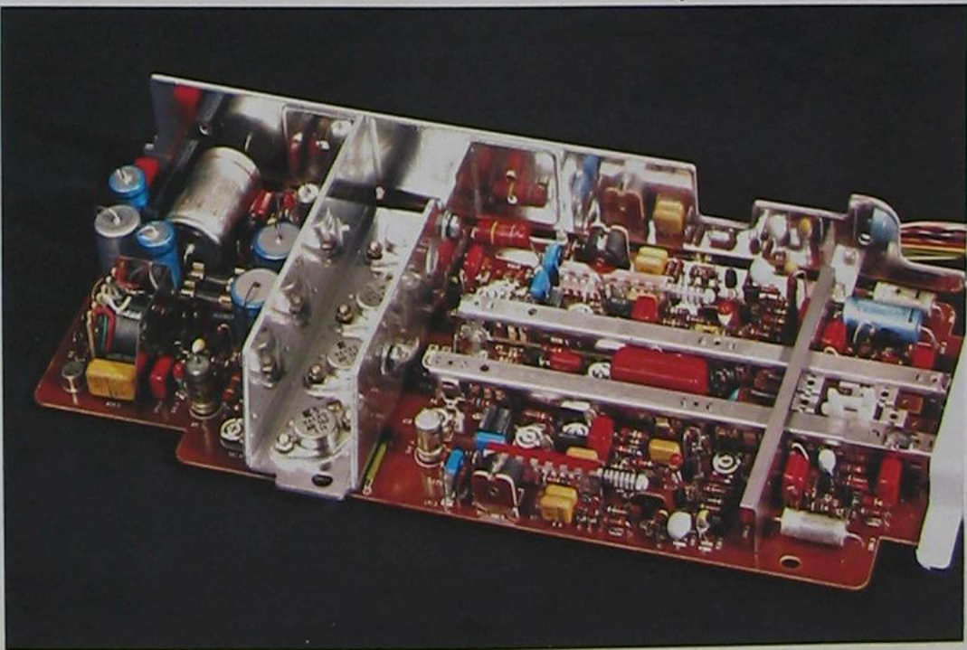
Das ist die Verstärkerplatte vom TK 240 HI-FI: modernste Technik klar und übersichtlich aufgebaut.
