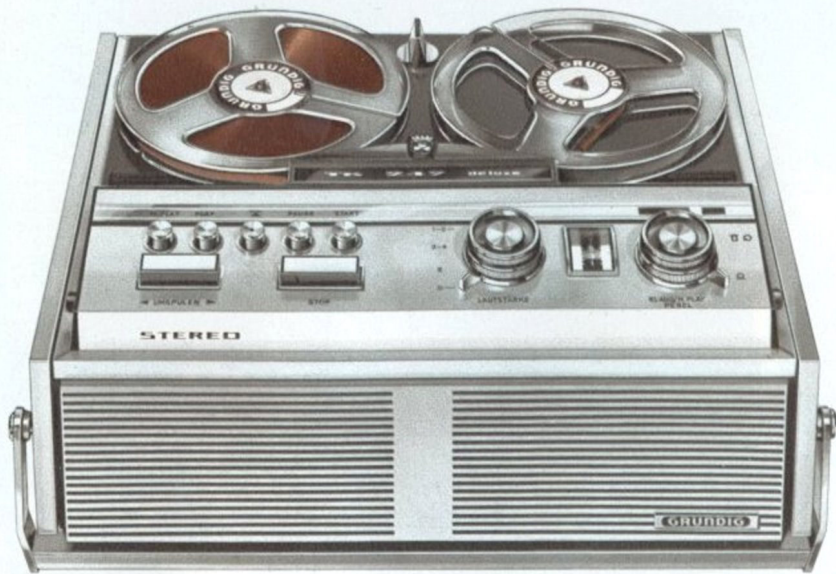
TK 247 de Luxe Stereo: Vollstereo-Tonbandgerät mit vier Superphon-Lautsprechern. Multiplayback, Mischregler, Geschwindigkeiten 9,5 und 19 cm/s
