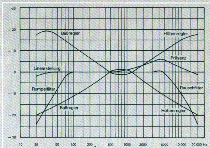
Frequenzgänge
