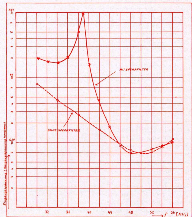
Abb. 2 Vorkreisselektion im Kanal 2 mit und ohne Sperrfilter
