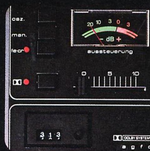
Elektronische Bandsortenschaltung und Aussteuerung. Elektronisch gesteuerte Band-Aufnahmeautomatik »AGFC«.
