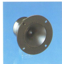
FH-10 Tweeter PA* Imp.: 8Ω fr.: 5-16kHz SPL: 99±2dB Pwr.,max: 50W min. Xov.: 6kHz weight: 320g
