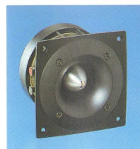
T-950 Tweeter PA-D* Imp.: 8Ω fr.: 2-20kHz SPL: 110±2dB Pwr.,max: 100W min. Xov.: 5kHz weight: 2250g
