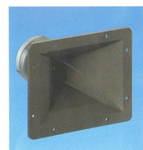
FH-300 Horn-Tweeter PA* Imp.: 8Ω fr.: 1.2-16kHz SPL: 106±2dB Pwr.,max: 120W min. Xov.: 2.5kHz weight: 990g
