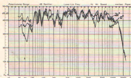
11 Sentry III, Einfluß der Hörwinkel 0°, 20° und 40° auf die Schalldruckkurve
