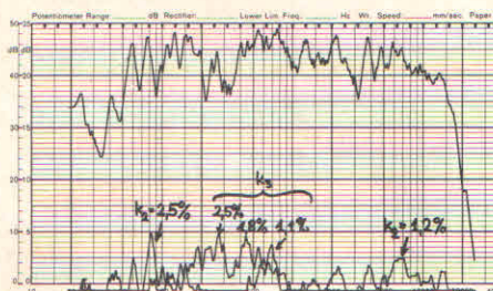
10 Sentry III, Schalldruckkurve, k_2 und k_3
