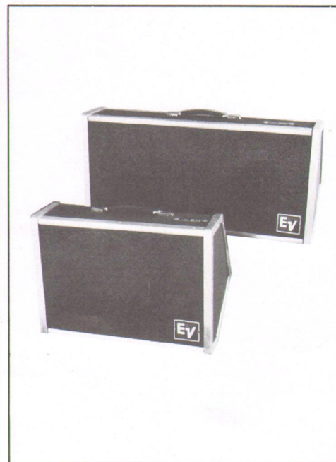
FM 12-2/FM 12-3 Monitor Systems. High efficient monitor systems using T35 tweeters and famous EVM 12L woofer. FM 12-3 also incorporates Thiele design vented midrange speaker. Edges are protected with aluminium trim. Hochwirkungsgrad Bühnenmonitore ausgerüstet mit T35 Hochtondruckkammertreiber und EVM 12L Basslautsprecher. FM 12-3 besitzt ebenfalls einen nach Thiele abgestimmten ventilierten Mitteltöner. Kanten durch Aluminiumprofil geschützt.
