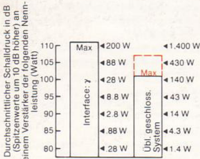
Interface γ erzeugt grösseren Schalldruck bei kleinerer Leistung als geschlossene Lautsprechersysteme.
