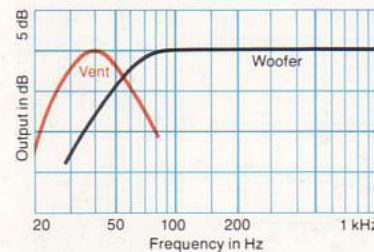
Der optimal ventilierte Interface-Lautsprecher. Die Öffnung wirkt als Tieftonlautsprecher, was die Basswiedergabe auf bemerkenswerte Weise verbessert.
