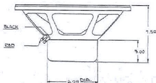
Fig. 1 - Dimensions
