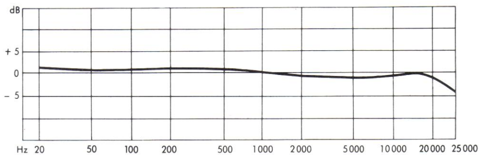
Frequenzkurve des ELAC STS 344-17 bezogen auf konstante Auslenkgeschwindigkeit.
