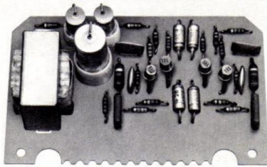
Transistor-Entzerrer-Vorverstärker PV 9
