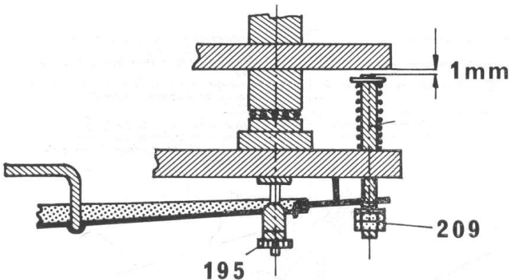
Fig. 10 Plattentellerbremse
