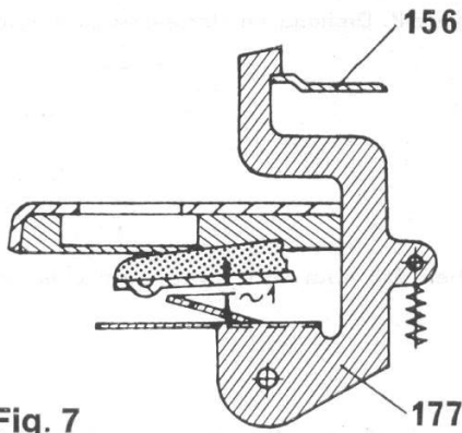
Fig. 7 Taststift-Einstellung
