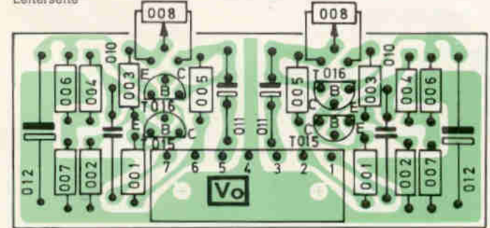
NF-Vorverstärkerplatine 02528 Leiterseite
