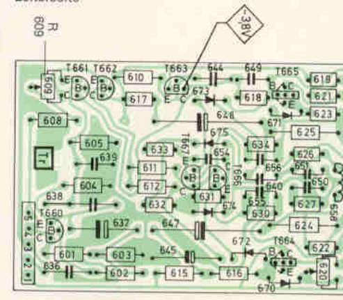
NF-Treiberplatte 02530 Leitersseite
