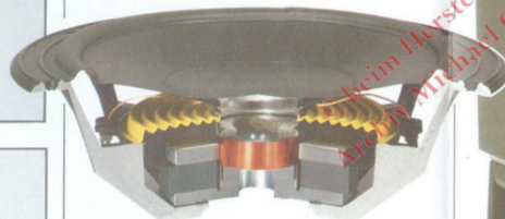
Schnitt durch den Baßlautsprecher der Compound 5
