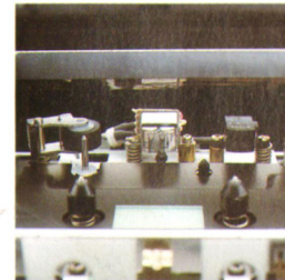
3-Kopf-Anordnung am Beispiel des HiFi-Cassetten decks Dual CC 8050.
