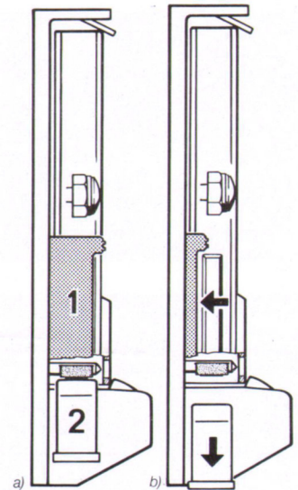
a) Cassette wird abgespielt. D.L.L.-Kontakte in Ruhestellung. Tonköpfe im Betriebszustand. b) Beim Greifen der Cassette schalten die Kontakte (1) der D.L.L.-Technik den Antrieb automatisch ab. Die Tonköpfe werden blitzschnell nach unten in Sicherheit gebracht (2).
