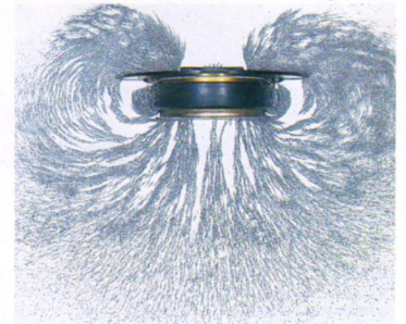
Ohne Feldlinien-Focussierung
