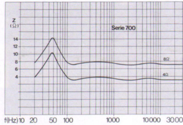
Der Verlauf der Impedanz Z in Abhängigkeit von der Frequenz f ist oberhalb der Eigenresonanz linear.
