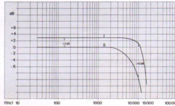
Das Reineisenband bringt bei richtiger Einstellung des Cassettendecks erheblichen Gewinn an Höhdynamik + 10 dB bei 10000 Hz und höheren Nutzpegel + 3 dB im übrigen Frequenzbereich. Kurve I: Reineisenband Kurve II: Chromdioxidband
