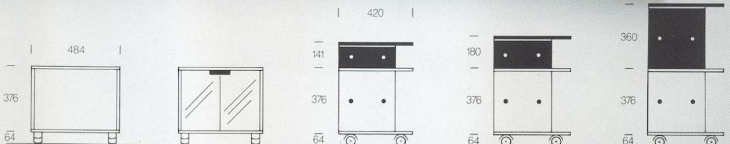
Grundelement 3000-1 mit 4 Rollen, elastischen Bändern und Halter für Kopfhörer.
