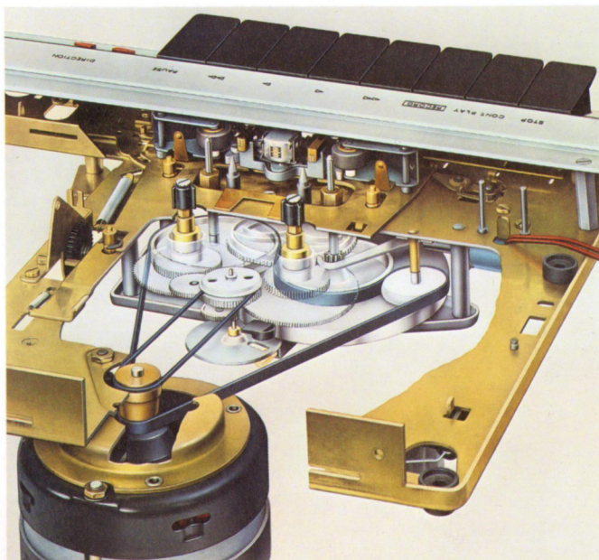
Dual Vierpol-Continuous-Pole-Motor mit getrenntem Antrieb von Tonwellen und Cassettenwickel.
