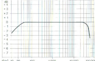
Leistungsbandbreite (k = 1%)
