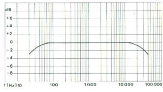
Leistungsbandbreite (k = 1%)
